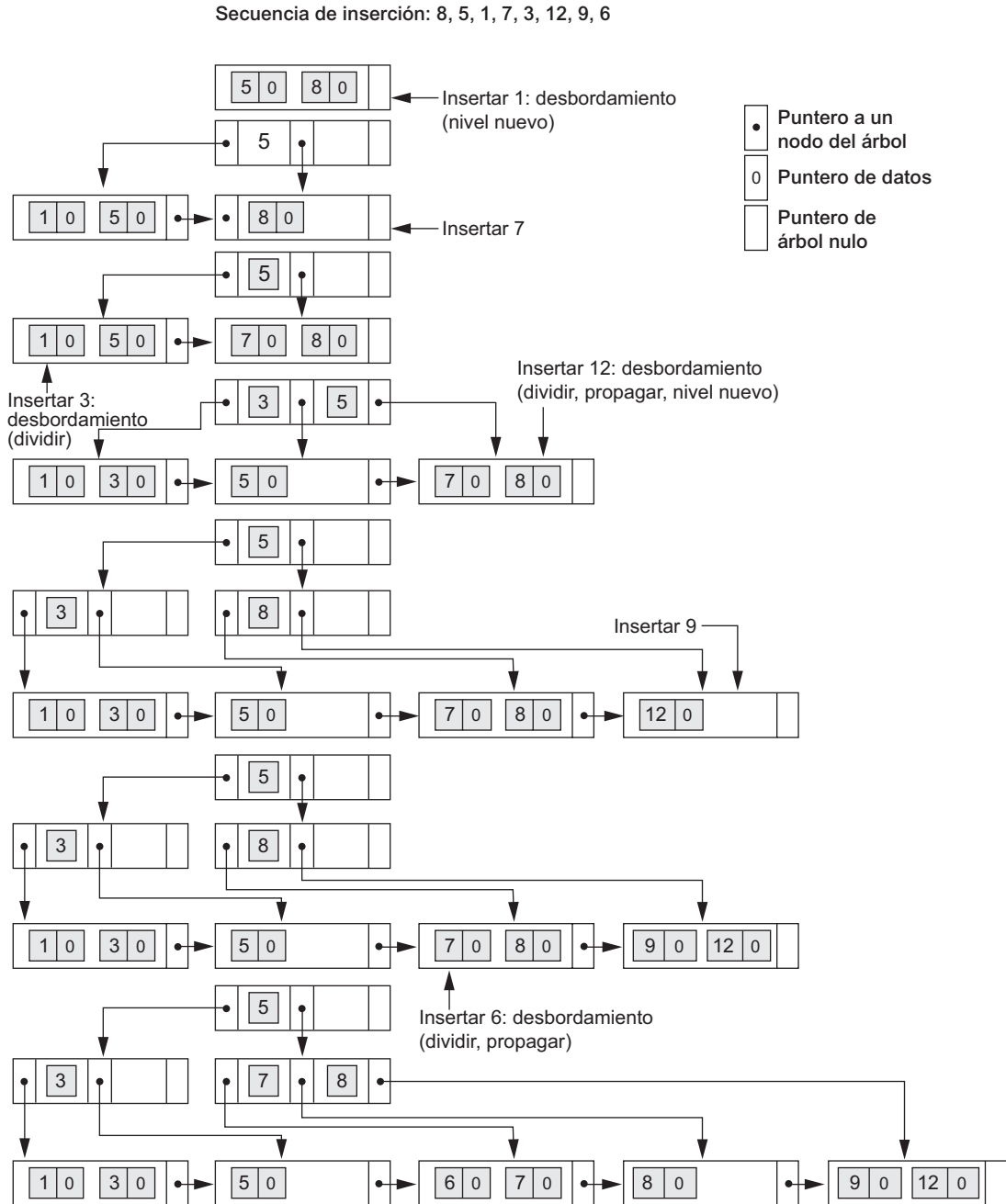
Figura 14.12. Ejemplo de inserción en un árbol B + con p = 3 y p_{hoja} = 2 .
