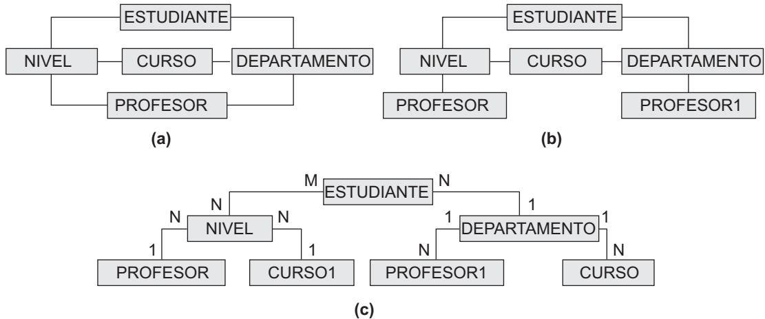
Figura 27.11. Conversión de un gráfico con ciclos en una estructura jerárquica (árbol).
